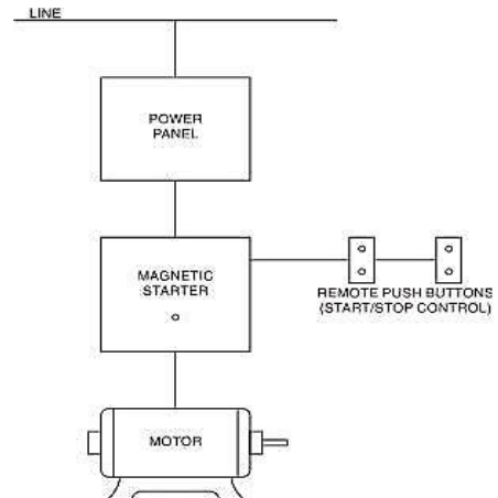
Motor wiring
