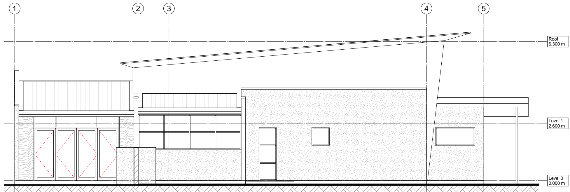
2 Elevation 2 - West A21 1:50
