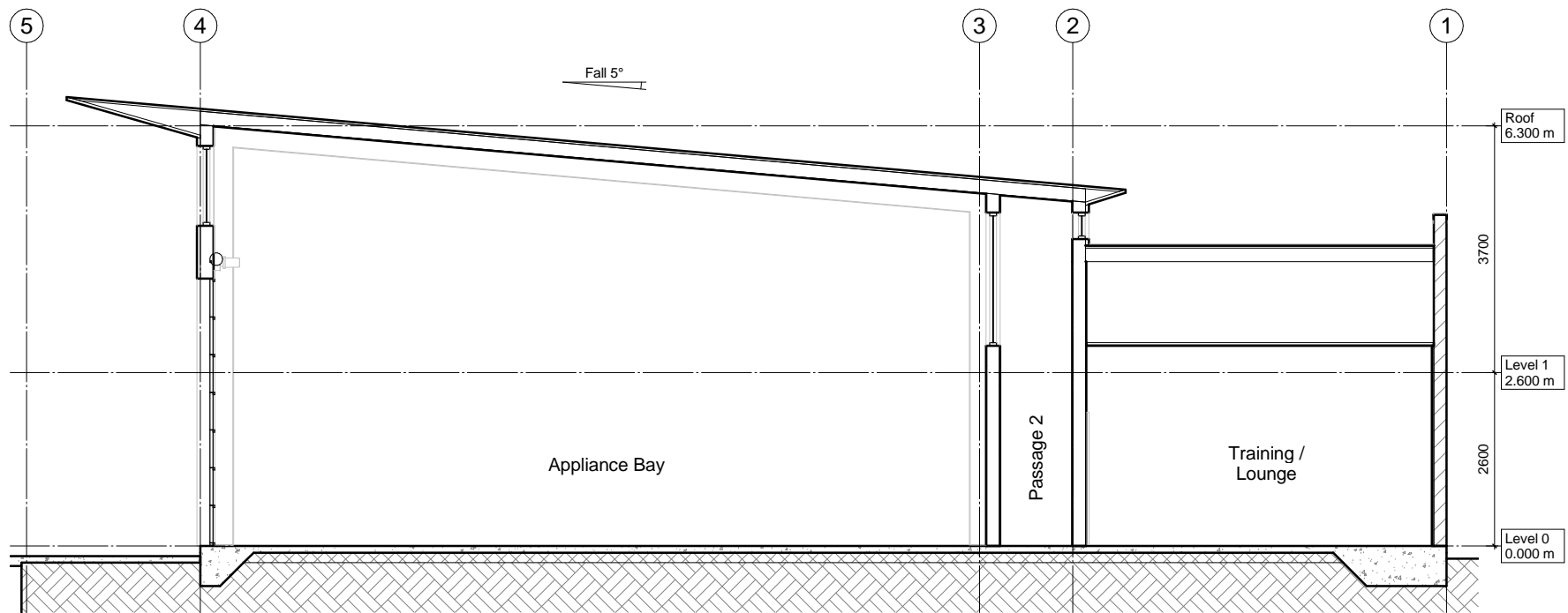
B Section B A21 1:50
