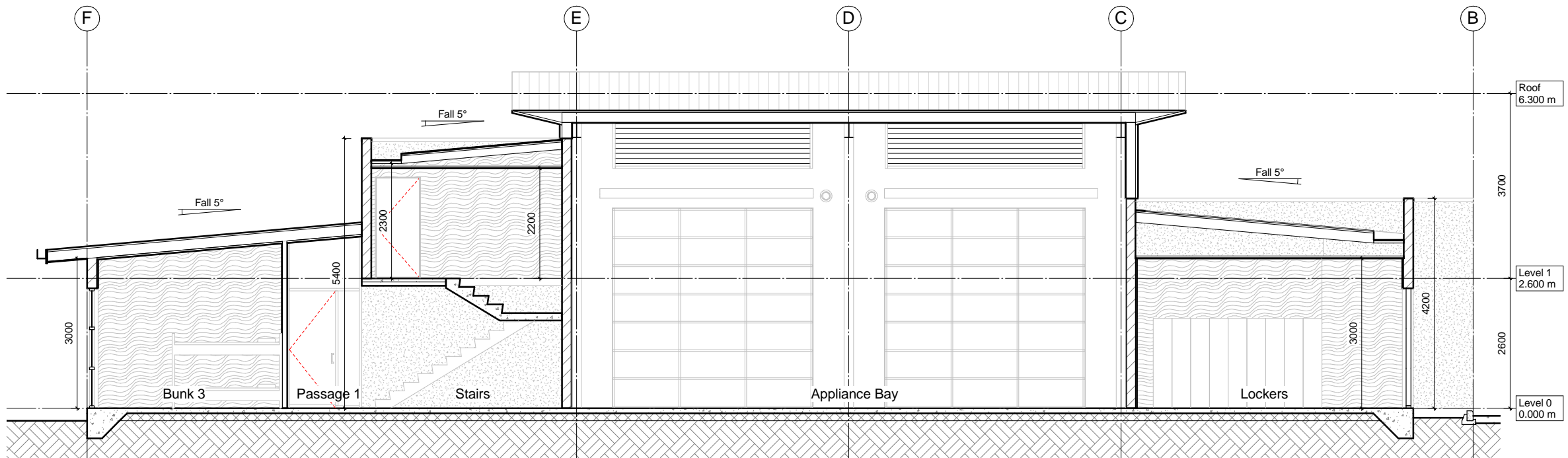
A Section A A21 1:50
